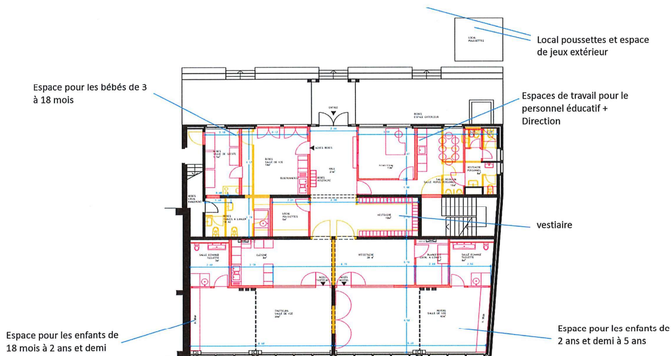
Fig. 1 Plan d'intention des locaux réaménagés
